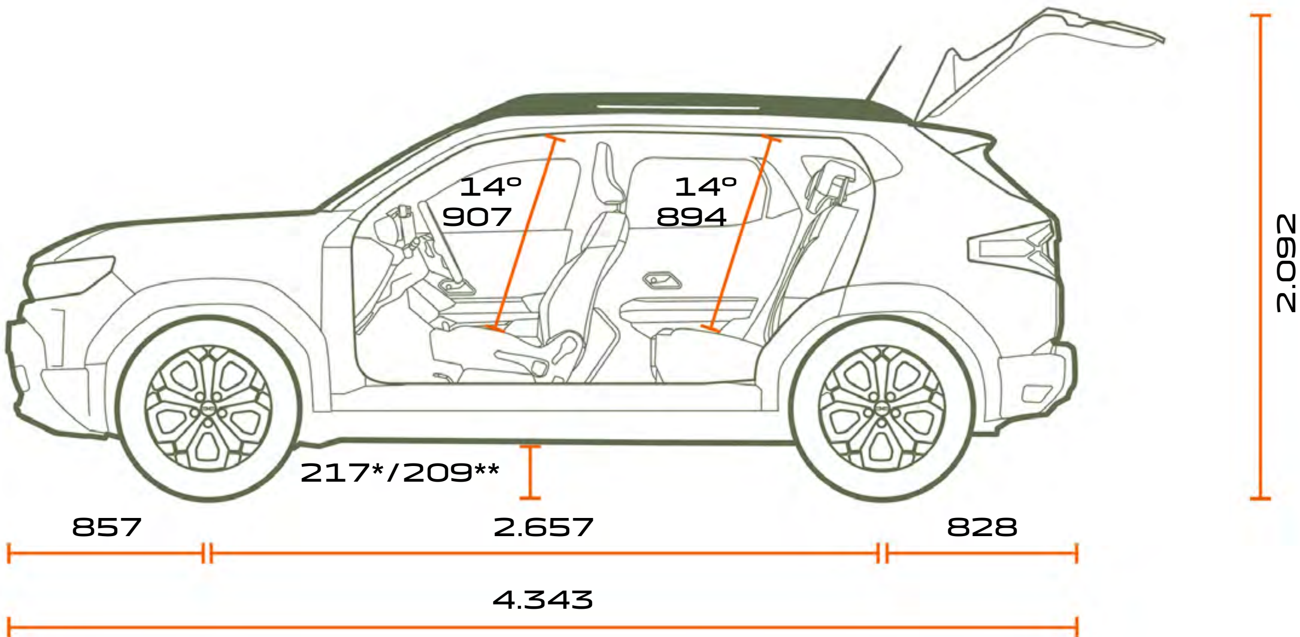
PROFILANSICHT
