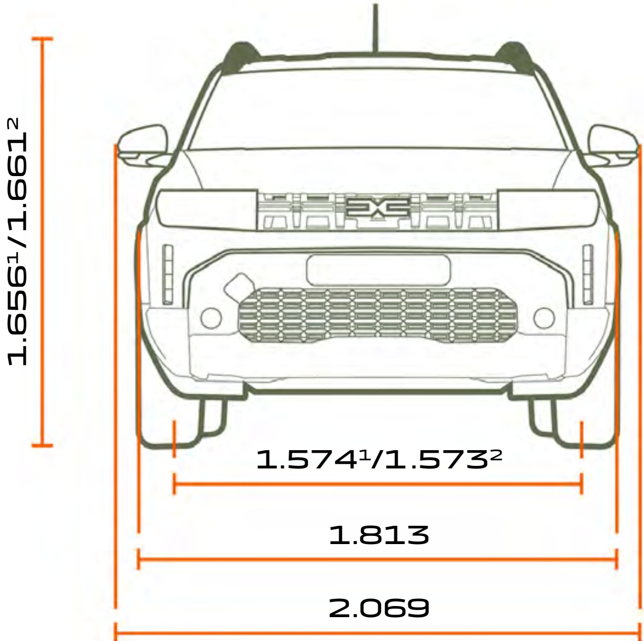
VORDERANSICHT
